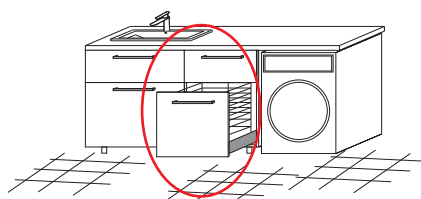
NEO-A/11, NEO-A/12 típusok beépített szennyestartó fiókja
