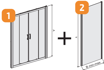
D4/TX5b zuhanyajtó - 1 db
