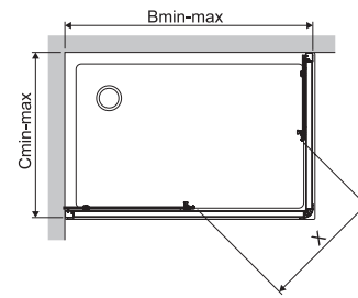
KNP/FREEZONE jobbos kivitel
